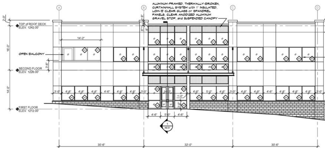
1 SOUTH ELEVATION A4.01 SCALE: 1/8" = 1'-0"
