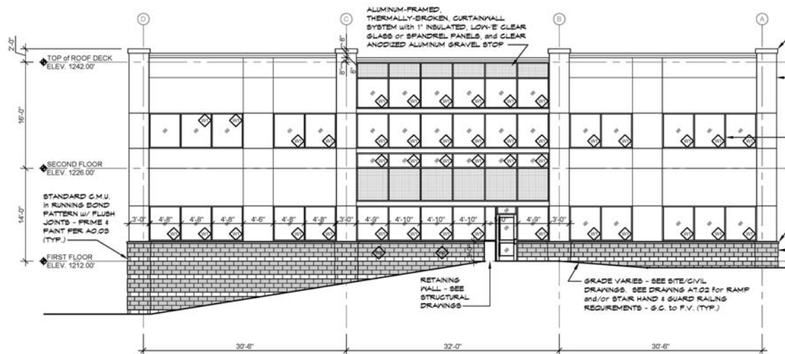
1 NORTH ELEVATION A4.02 SCALE: 1/8" = 1'-0"
