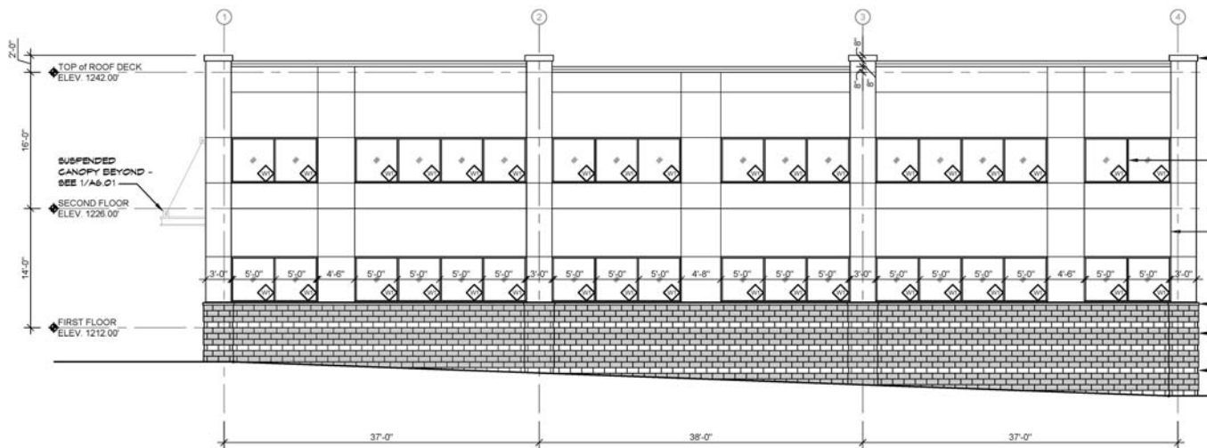
2 EAST ELEVATION A4.02 SCALE: 1/8" = 1'-0"
