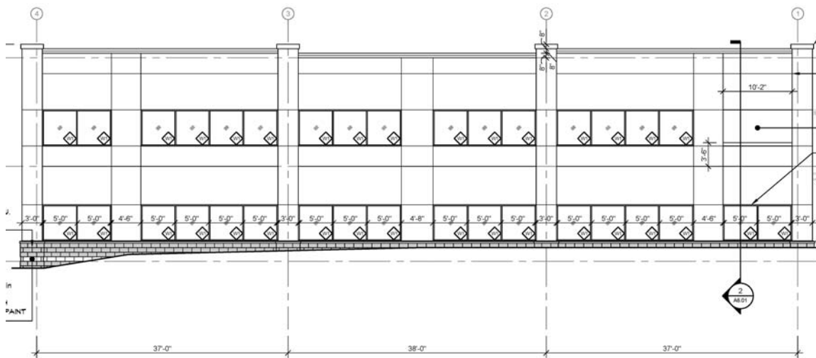
2 WEST ELEVATION A4.01 SCALE: 1/8" = 1'-0"
